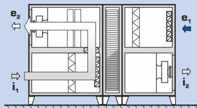
Umluftheizung oder -kühlung
