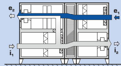
Kombinierte Lüftung (Umluftbetrieb)
