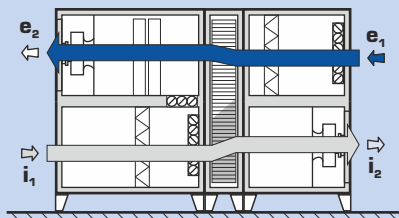
Lüftung mit Wärmerückgewinnung und Nacherwärmung (oder Kühlung)
