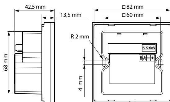
Unterputzdose
