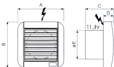
Abmessungen (mm)
